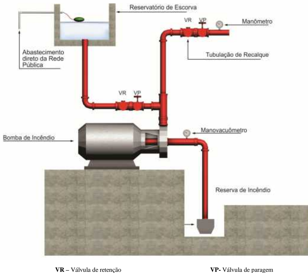
Figura C.3 – Exemplo de afogamento de bomba de incêndio
